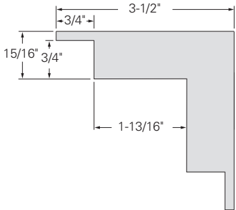
KLEER KONCEAL® CORNER
